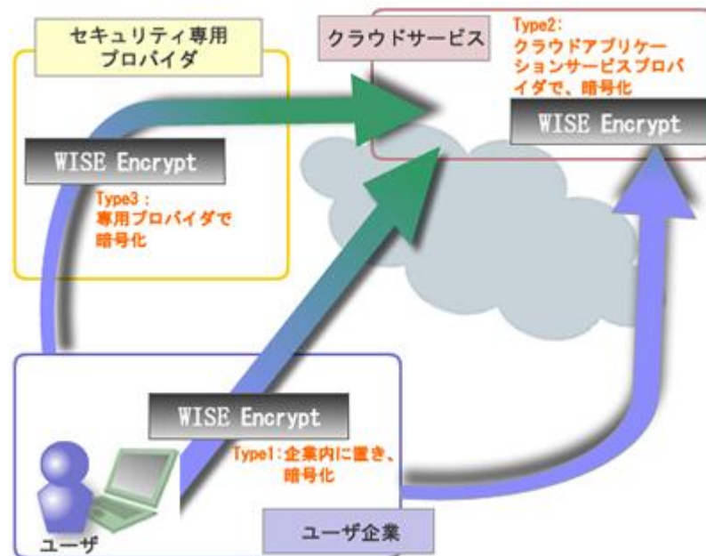
WISE Encryptの導入利用形態
